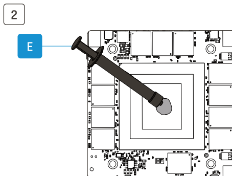
DE Wärmeleitpaste auftragen
