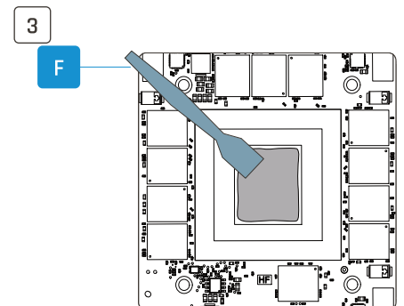
FR Appliquer la pâte thermique
