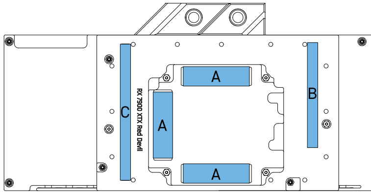
DE Wärmeleitpads auf dem Kühlblock platzieren
